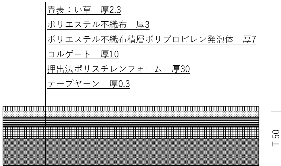
畳の断面詳細図
