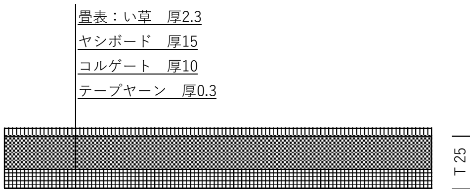
畳の詳細断面図
