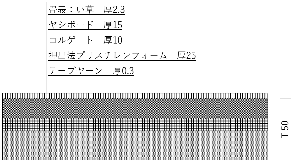
畳の断面詳細図
