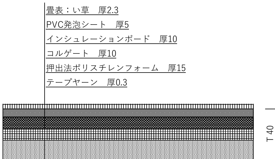
畳の断面詳細図
